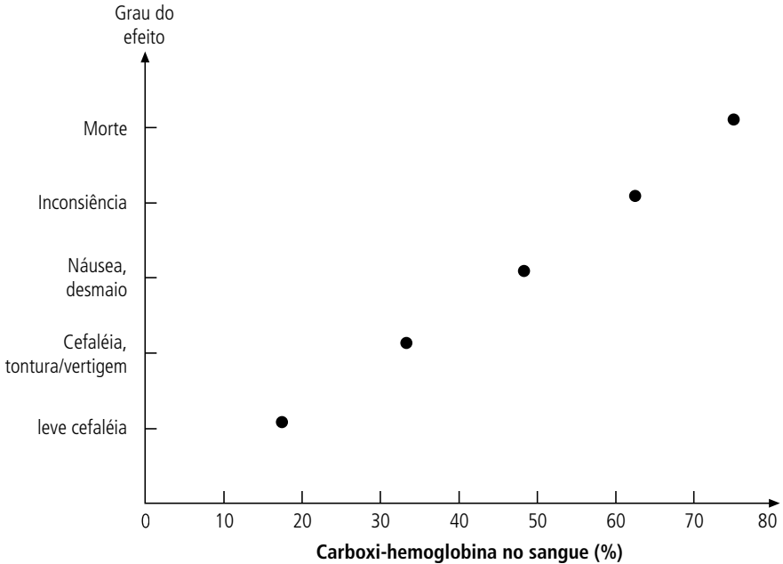
Figura 9.5. Relação dose-efeito
